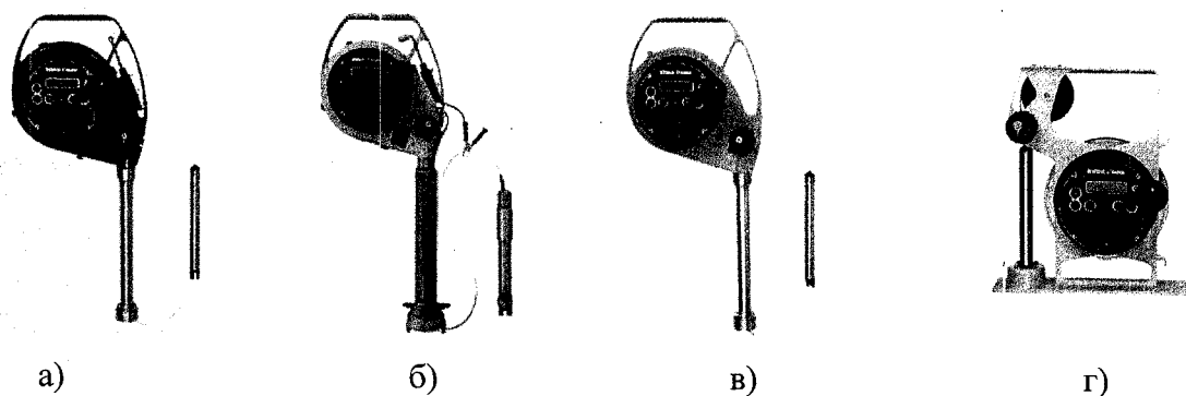
Р и с у н о к 1 – Уровнемеры электронные переносные HERMetic UTImeter а) Gtex; б) Gtex2000; в) Rtex; г) Otex.
